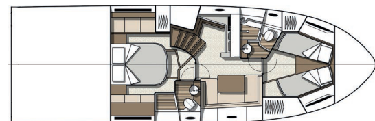
LOWER DECK PONT INFÉRIEUR
