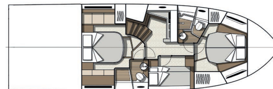
LOWER DECK WITH 3 rd OPTIONAL CABIN PONT INFÉRIEUR AVEC 3 ème CABINE OPTIONNELLE
